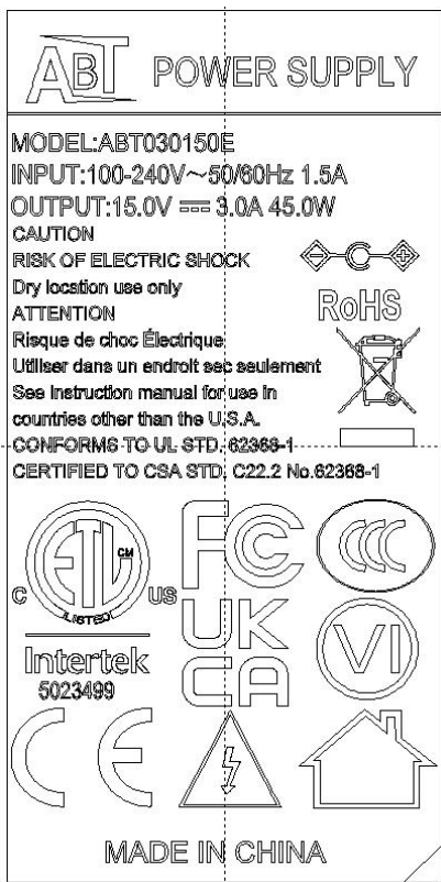
铭板内容
